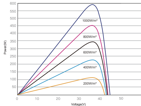
昊宇光伏P-V曲线图(595W)
