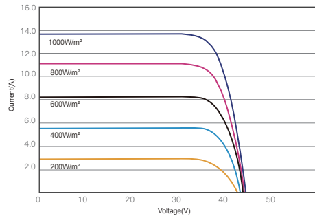
昊宇光伏I-V曲线图(595W)
