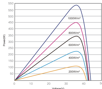
昊宇光伏P-V曲线图(590W)
