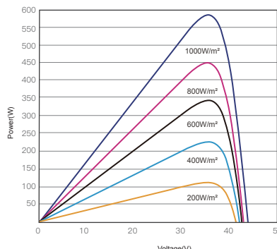
昊宇光伏功率-电压曲线图(590W)
