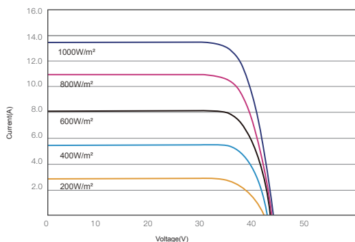
昊宇光伏电流-电压曲线图(590W)
