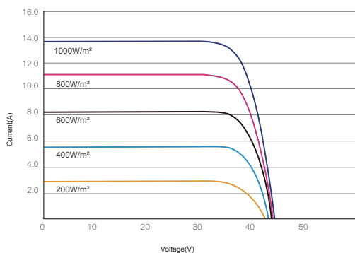
昊宇光伏电流-电压曲线图(575W)
