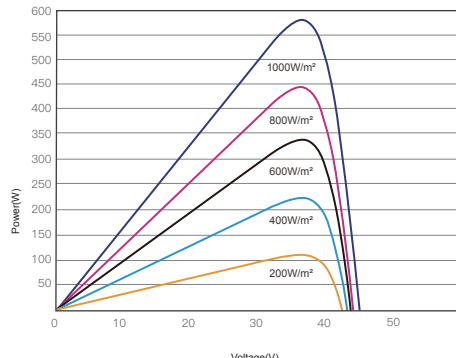
昊宇光伏功率-电压曲线图(575W)
