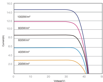
昊宇光伏电流-电压曲线图(595W)
