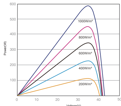
昊宇光伏功率-电压曲线图(595W)
