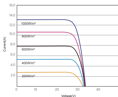
昊宇光伏电流-电压曲线图(425W)
