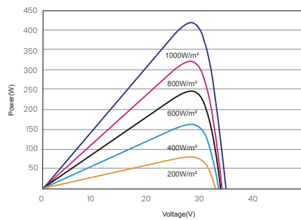
昊宇光伏功率-电压曲线图(425W)
